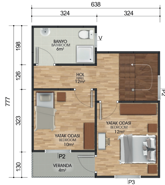
1. Kat Planı / First Floor Plan 41 m 2 + 4 m 2 = 45 m 2
