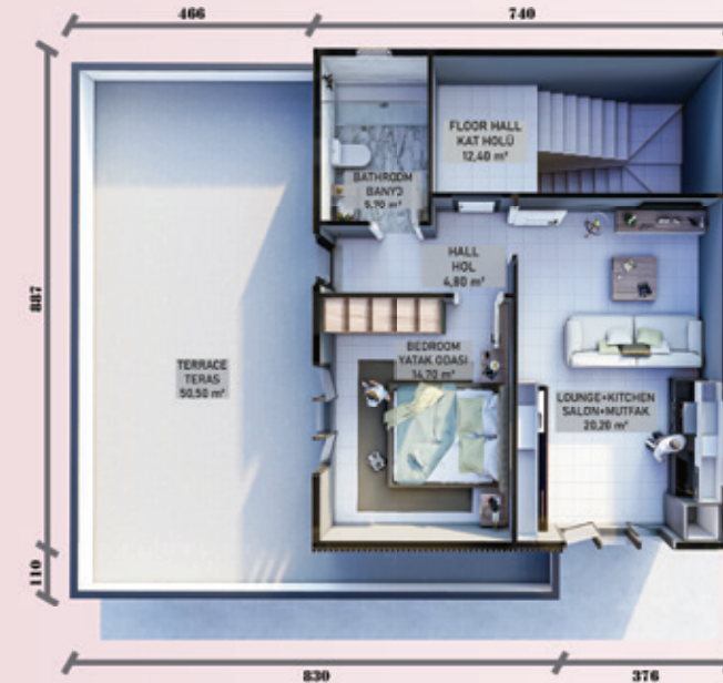
1. KAT PLANI
